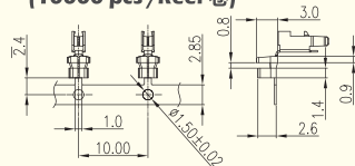
小電源/剎車壓接母針 Mini Power/Brake Crimp Socket XC-MC-7S-10K (10000 pcs /Reel 卷)
