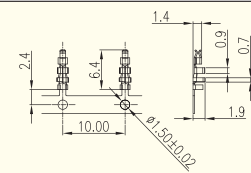
小電源/剎車壓接母針 Mini Power/Brake Crimp Socket XC-MC-7S-10K (10000 pcs /Reel 卷)
